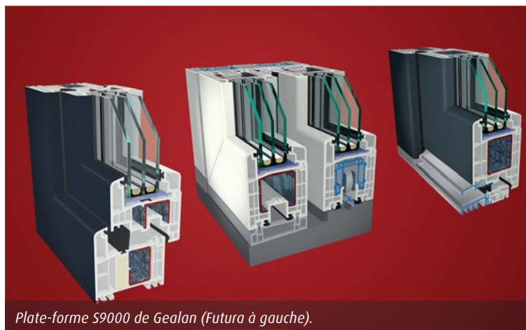
Version Design du couissant levant S 9000 de Gealan, plaxage AnTeak.
