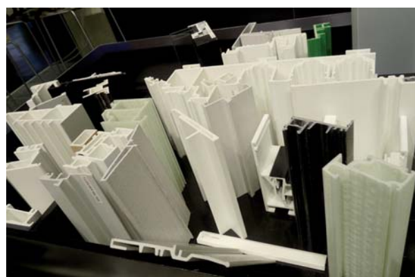
Profilés composites réalisés sur mesure pour ses clients par Fiberline Composites.
