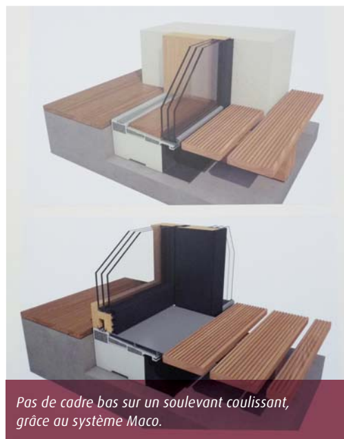
Prolongement de seuil PMR extérieure. Maco.
