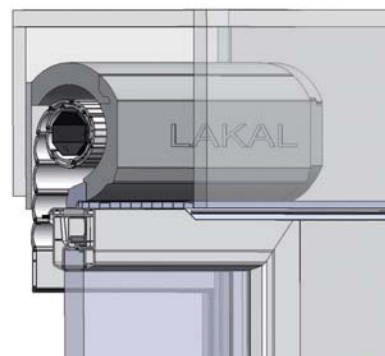
IsoProtect3, caisson de volet roulant isolé. Lakal.
